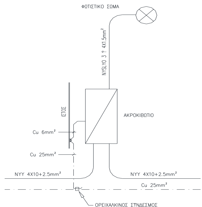
ΔΙΑΓΡΑΜΜΑ ΣΤ'ΝΔΕΣΜΟΛΟΓΙΑΣ ΦΩΤΙΣΤΙΚΟΥ
