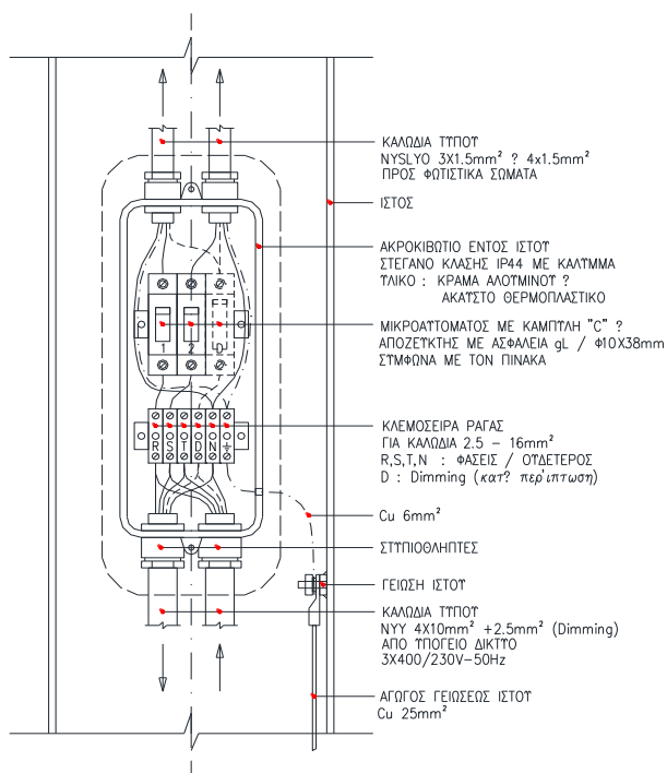
ΔΙΑΤΑΞΗ ΑΚΡΟΚΙΒΩΤΙΟ ΙΣΤΟΥ
